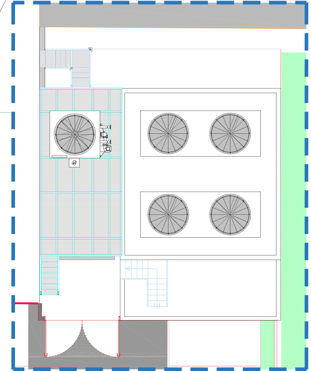
ZONA DI INTERVENTO STATO FUTURO - SCALA 1:100
