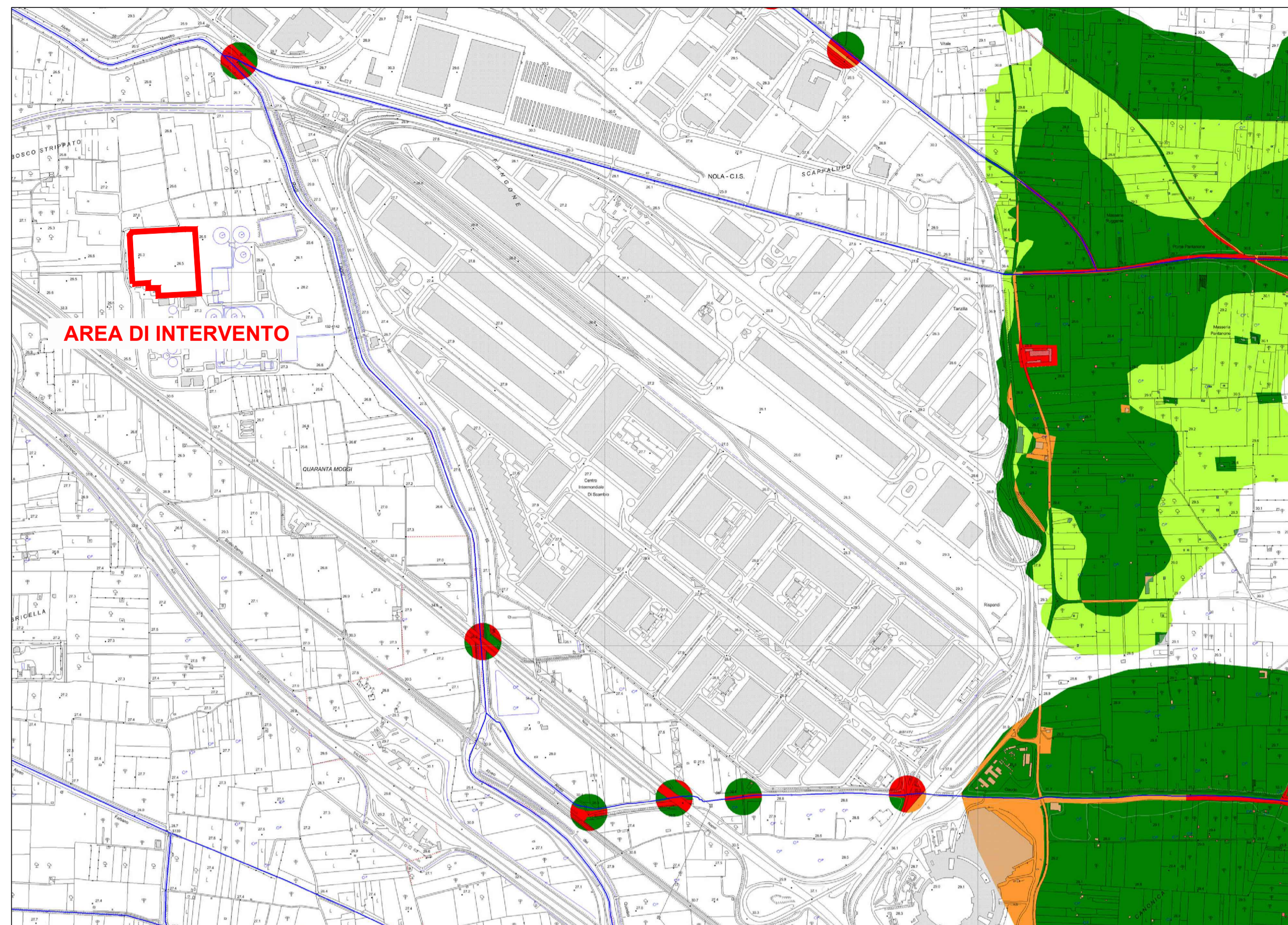
Carta del rischio idraulico - RI448022 - SCALA 1: 10.000
