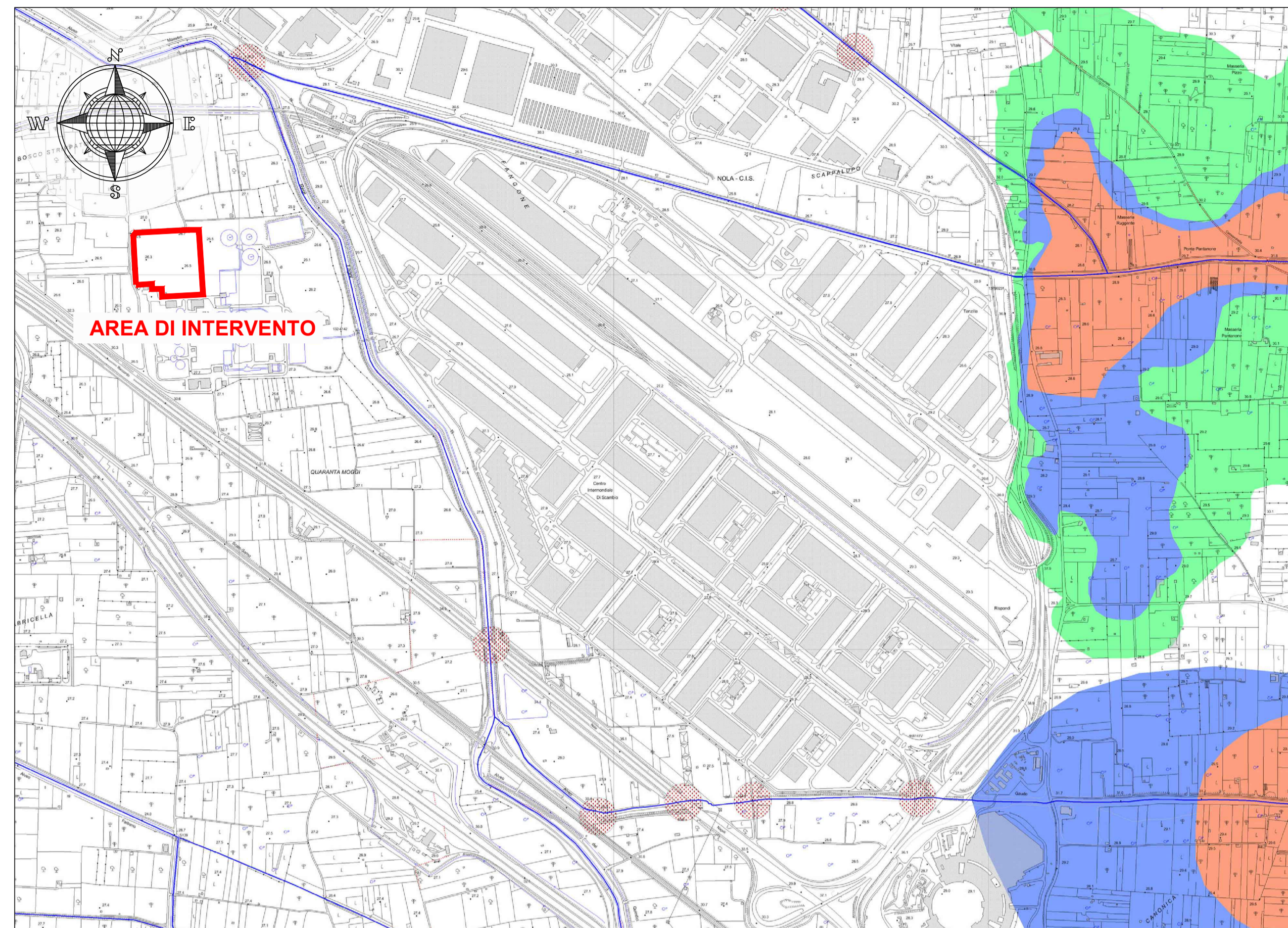
Carta della pericolosità idraulica - PI448022 - SCALA 1: 10.000
