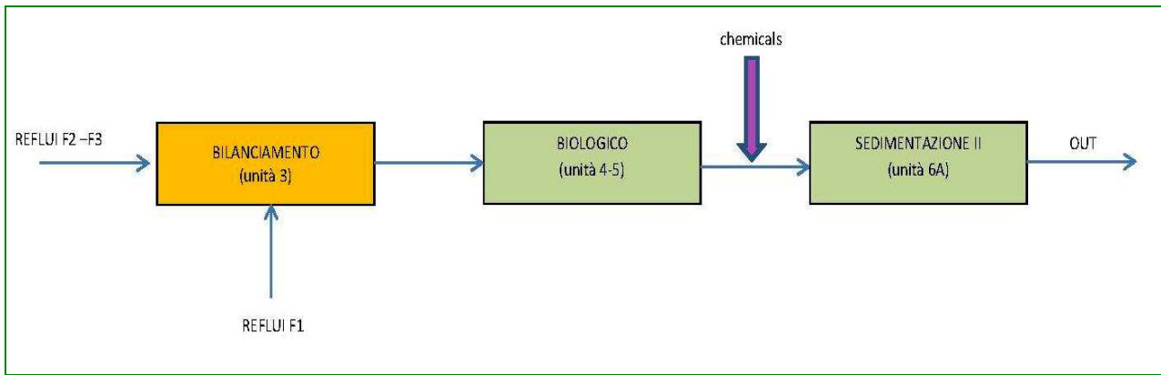
Schema semplificato del processo impianto F2
