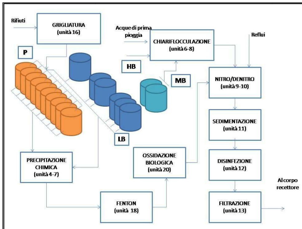
Figura 1 – Schema a blocchi processo di trattamento
