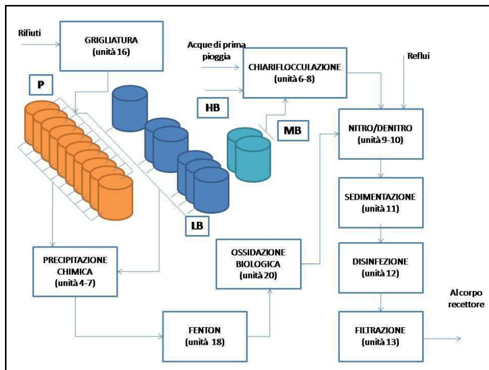
Figura 2.1 - Schema semplificato del processo depurativo
