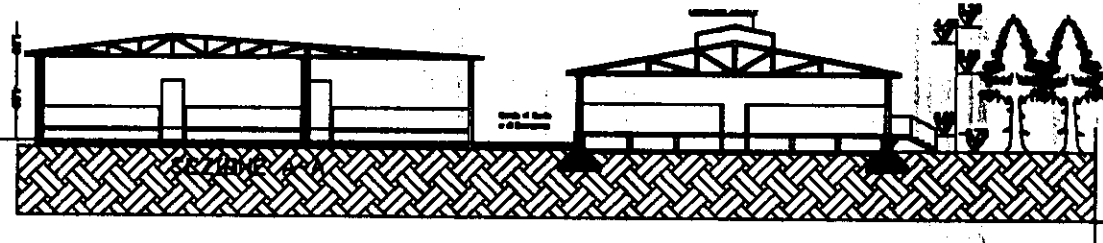
SEZIONE A-A
